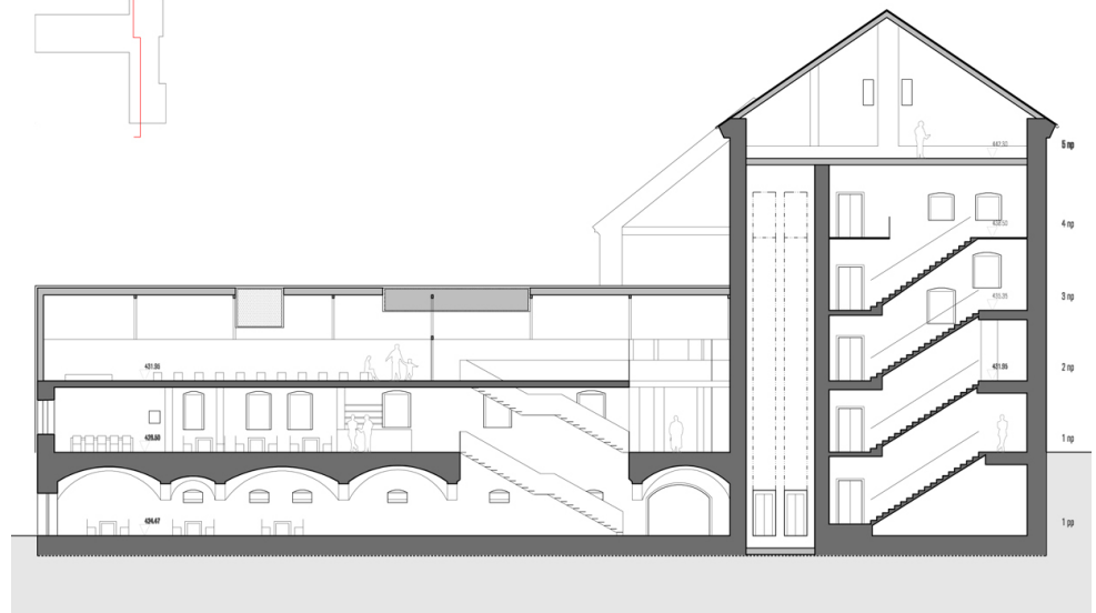
Coupe d'extension
