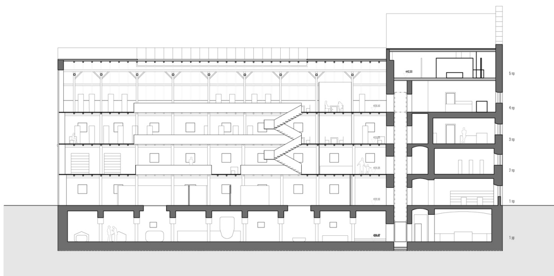
Coupe bibliothèque
